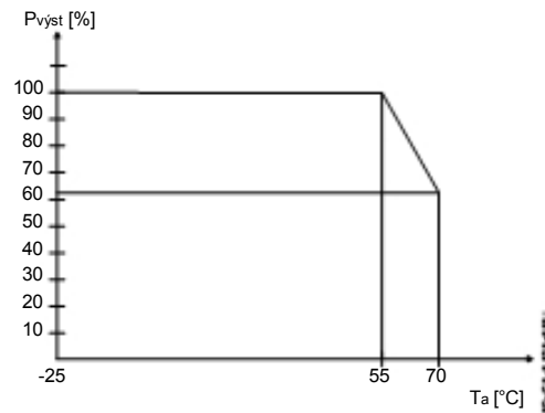
Obr. 5 Snížení zatížitelnosti
